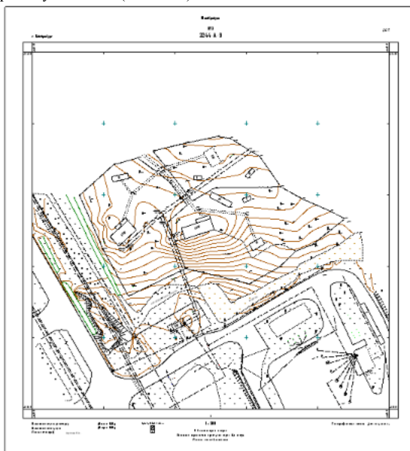
Рис. 4.89. Чертежная модель планшета
