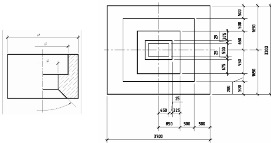
Рис. 7 Нанесение размеров на чертежах симметричных изделий
