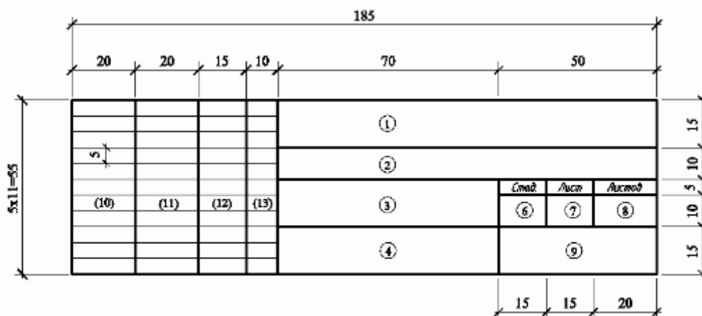
Рис.2. Основная надпись на листах чертежей зданий
