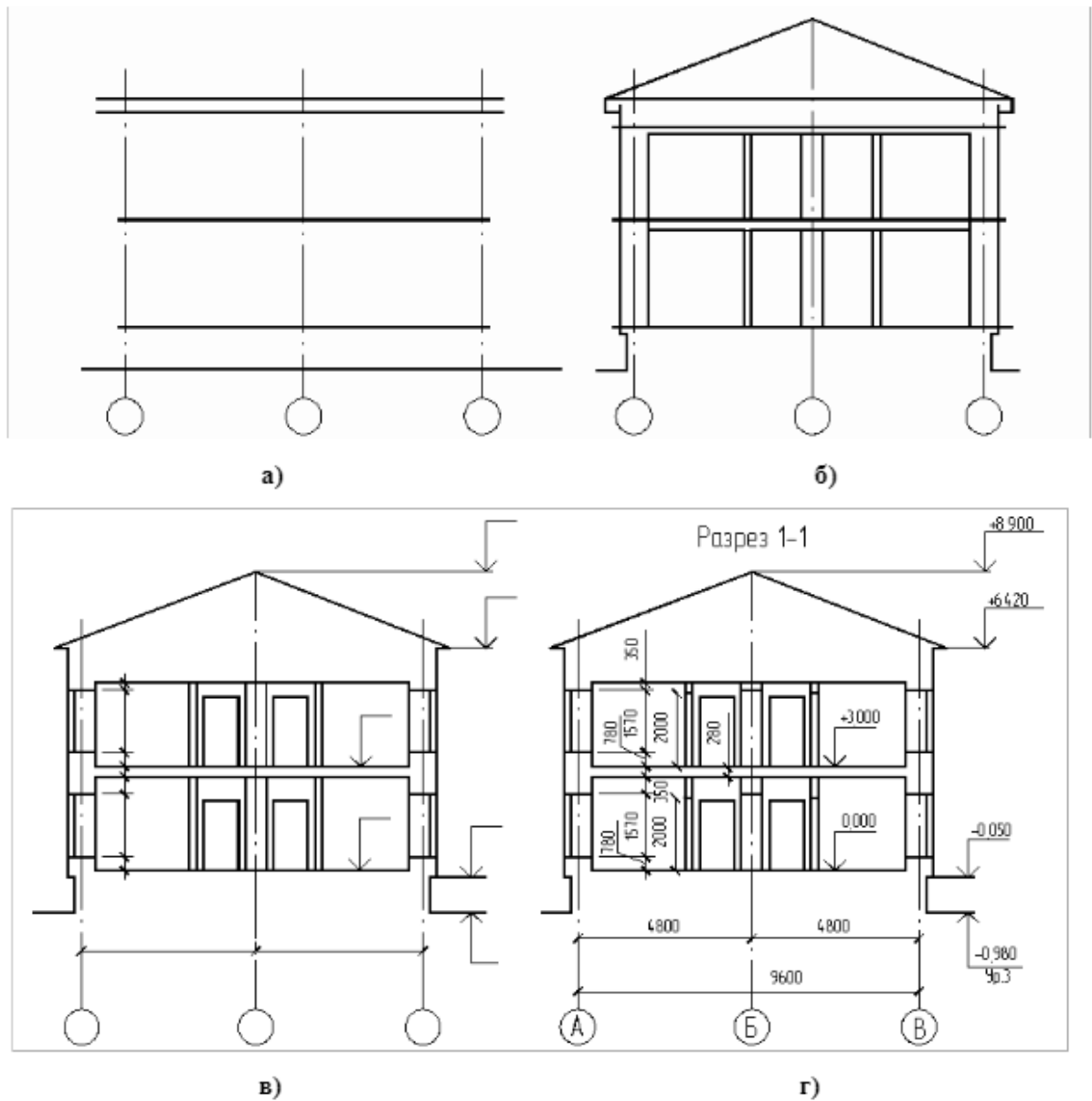
Рис. 15. Последовательность вычерчивания разреза.
