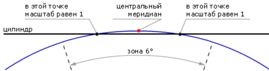
Рис.1.8. Проекция UTM
