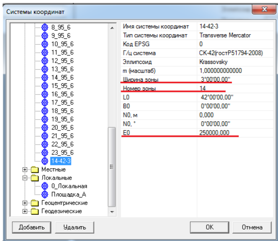
Рис.1.9. Создание системы координат 14 трехградусной зоны
